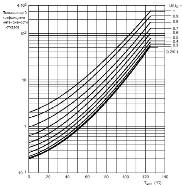
Рис. 5. Повышающие коэффициенты интенсивности отказов (справочник MIL HDBK-217F)
