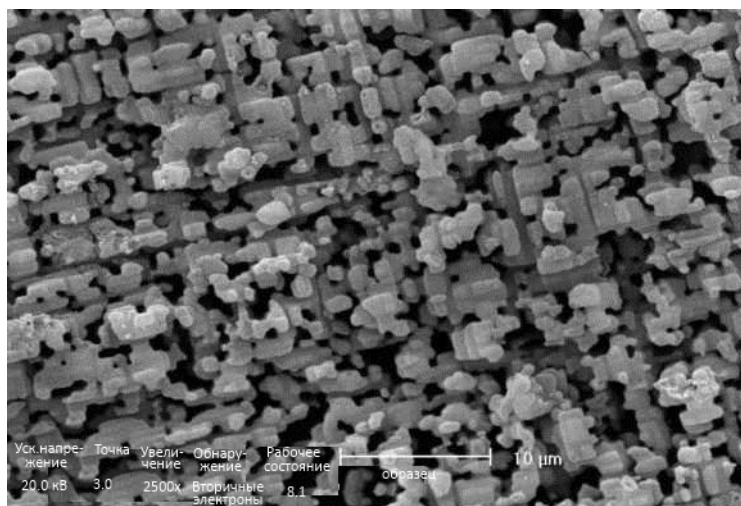
Рис. 2. Протравленная анодная фольга. Вид сверху
